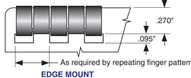
EDGE MOUNT
